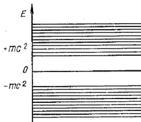
Рис. 2. Уровни с отрицательными значениями энергии
