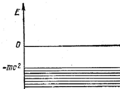
Рис. 2. Уровни с отрицательными значениями энергии
